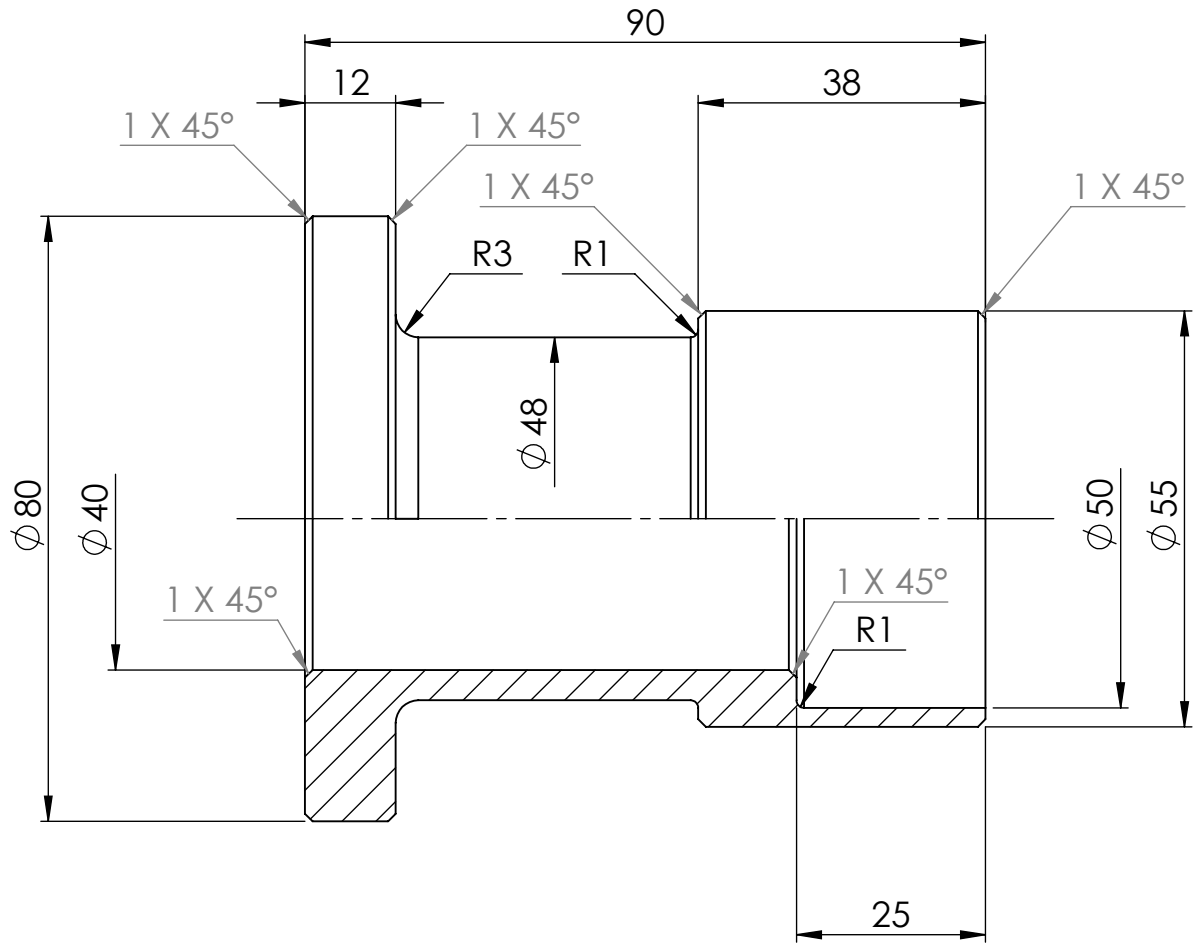
SECTION A-A
